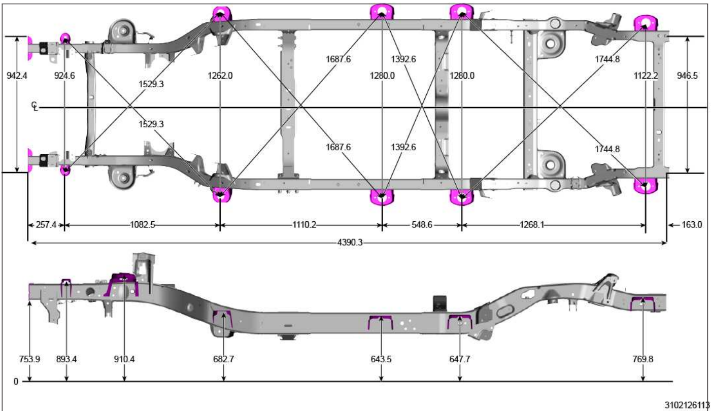
Frame Dimensions- 4 Door
