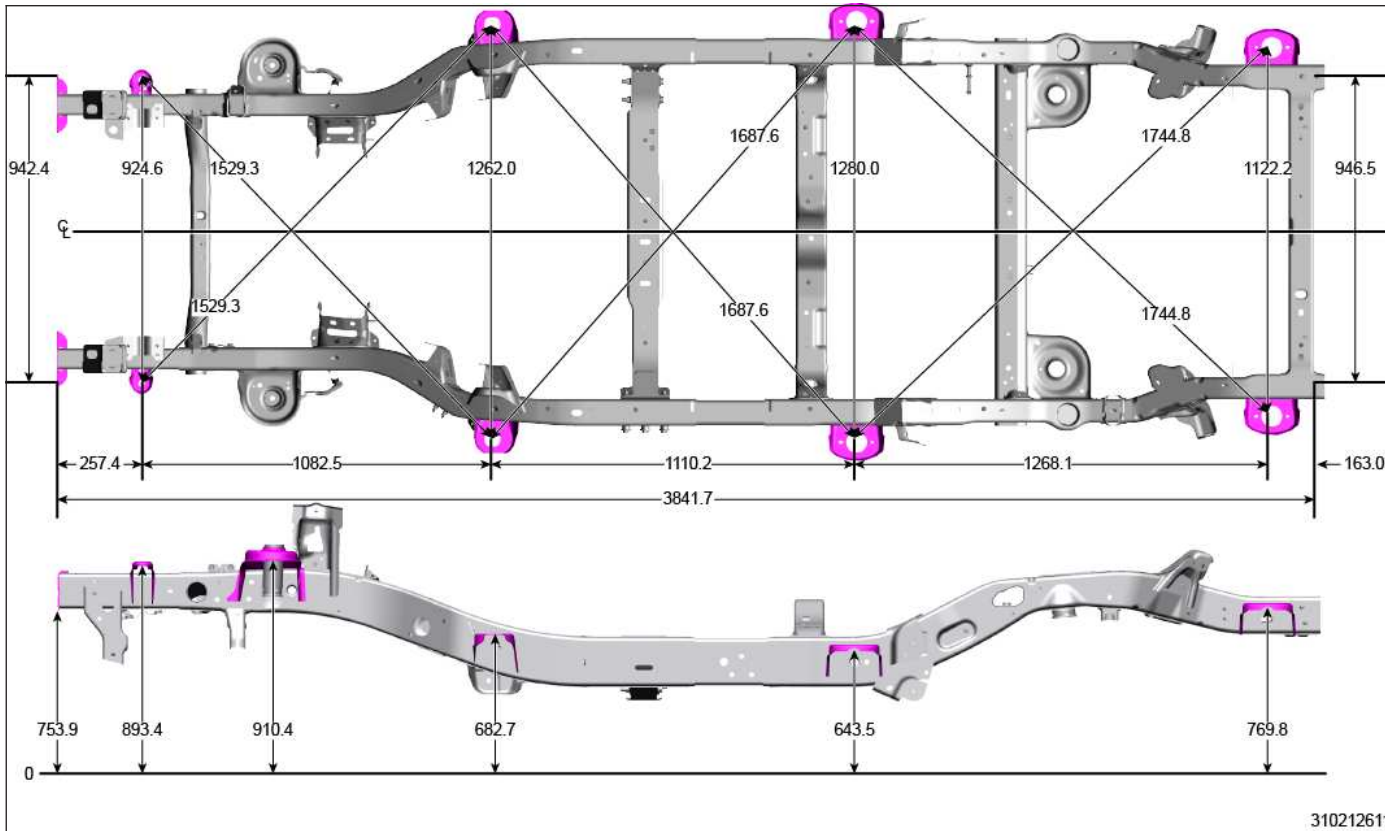
Frame Dimensions- 2 Door (JL 74)
